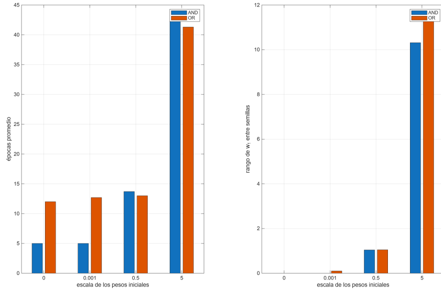
Figura 2: Efecto de la escala de los pesos iniciales en el Perceptrón. A la izquierda las épocas promedio hasta converger y a la derecha la dispersión de los pesos finales entre semillas
