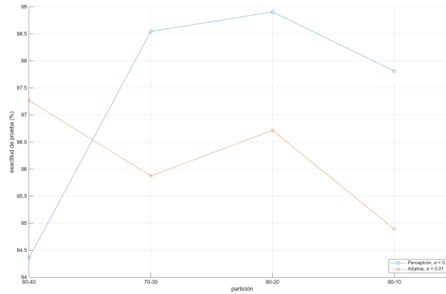
Figura 5: Exactitud sobre el conjunto de prueba de los dos modelos según la proporción de partición
