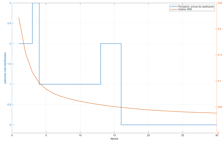
Figura 4: Dinámica del error sobre la compuerta AND de dos entradas. El eje izquierdo cuenta los patrones mal clasificados por el Perceptrón y el derecho mide el MSE del Adaline
