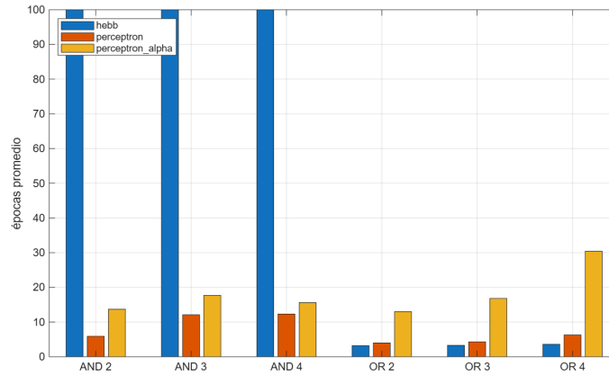
Figura 1: Épocas promedio hasta la convergencia con las tres reglas de ajuste. Las barras de la regla hebbiana en AND alcanzan el tope de cien épocas porque nunca convergen
