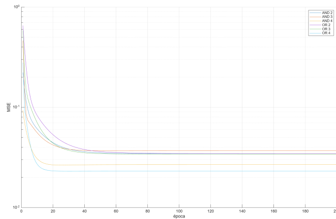
Figura 3: Curva de error de entrenamiento del Adaline sobre las seis compuertas con la tasa de aprendizaje base. La escala vertical es logarítmica
